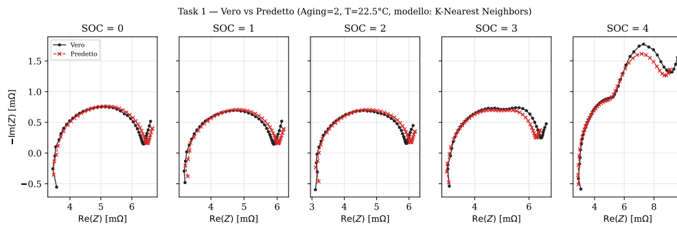
Figura 5.2: Curve previste (rosso, tratteggiate) sovrapposte alle vere (nero) per la coppia ( Aging = 2, T = 22.5^\circ\text{C} ) esclusa, una per ciascuno dei 5 livelli di SOC. Il modello vincente (KNN distance-weighted) ricostruisce semicerchio e coda diffusiva con errore inferiore al millesimo di milliohm.
