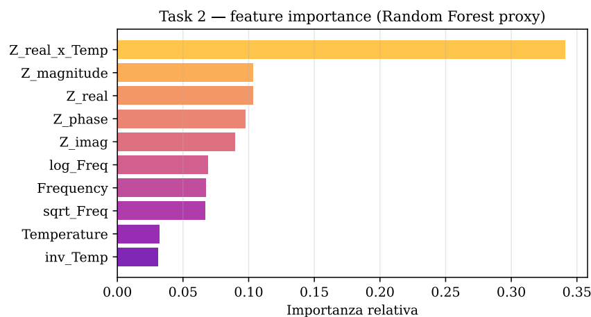
Figura 6.4: Feature importance restituita dal Random Forest (proxy interpretabile dell'SVM-RBF). L'interazione \text{Re}(Z) \times T domina la classifica.
