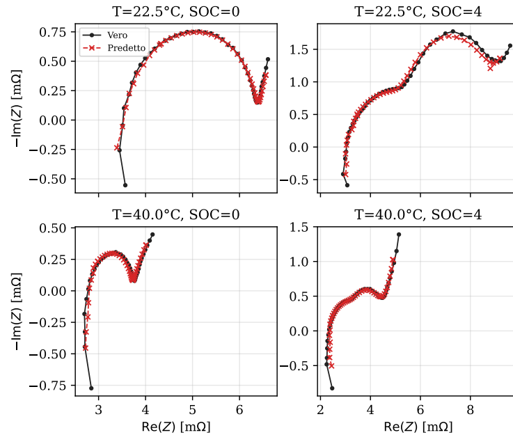
Figura 7.3: Quattro curve di Nyquist riconcostruite (rosso) sovrapposte alle vere (nero), prese a due temperature e due SOC diversi. Pur non avendo mai osservato \text{Aging} = 2 in addestramento, il modello ricostruisce correttamente sia il semicerchio sia la coda diffusiva.
