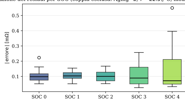
Figura 5.3: Distribuzione dei residui assoluti |\hat{Z} - Z| per ciascuno dei 5 SOC, sulla coppia esclusa ( Aging = 2, T = 22.5^\circ C ). Le mediane sono concentrate sotto la dispersione fisiologica delle misure ( \sim 1 \text{ m}\Omega ); i SOC estremi (0 e 4) hanno una coda leggermente più lunga, coerentemente con la maggior curvatura del Nyquist a quegli stati di carica.
