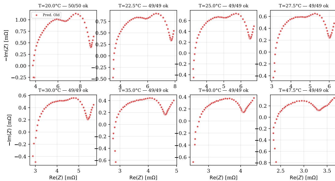
Figura 6.3: Le 8 curve di Nyquist della coppia esclusa ( Aging = 4, SOC = 3 ) – una per temperatura – con i punti colorati dalla classe predetta dall'SVM-RBF (blu = Young, rosso = Old). La classe vera è Old : tutte le 8 curve sono interamente classificate rosse, alle 8 diverse temperature.
