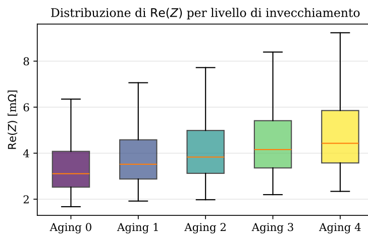
Figura 3.3: Distribuzione di \text{Re}(Z) stratificata per livello di Aging, aggregata su tutte le temperature, SOC e frequenze. La mediana sale monotonamente con l'invecchiamento.
