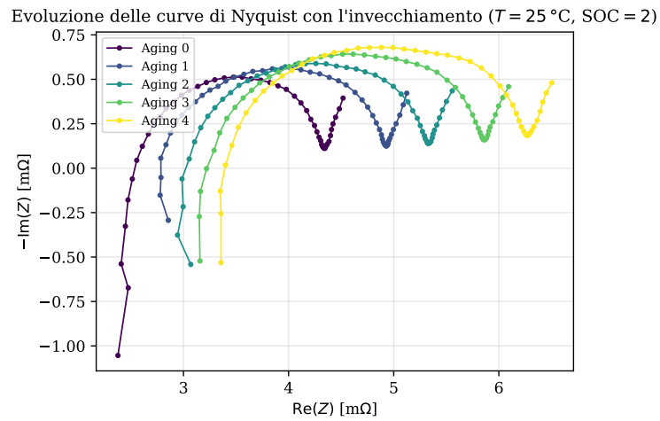
Figura 3.2: Evoluzione delle curve di Nyquist con il livello di invecchiamento, a T = 25\text{ }^{\circ}\text{C} e \text{SOC} = 2 . Il semicerchio si allarga e la coda si trasla a destra al crescere dell'Aging – giustificazione empirica della separabilità che il Task 2 sfrutterà.
