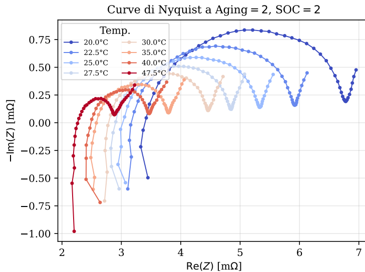
Figura 3.1: Curve di Nyquist al livello di invecchiamento centrale ( Aging = 2 , SOC = 2 ) per le otto temperature del dataset. La forma a semicerchio + coda diffusiva è la firma elettrochimica della cella; cresce in ampiezza al diminuire della temperatura.
