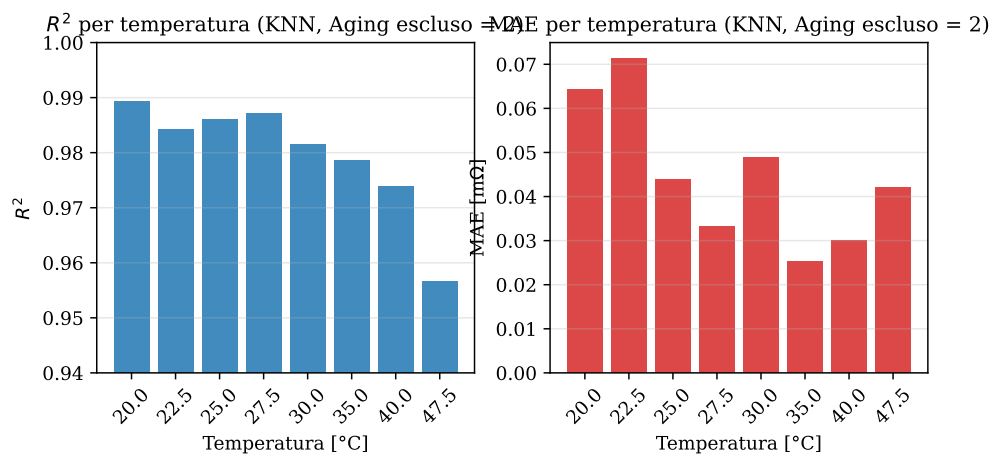
Figura 7.2: R^2 e MAE per livello di temperatura del modello KNN vincitore. La performance degrada al bordo superiore della finestra termica (47.5 °C, R^2 = 0.957 ) per effetto di boundary .
