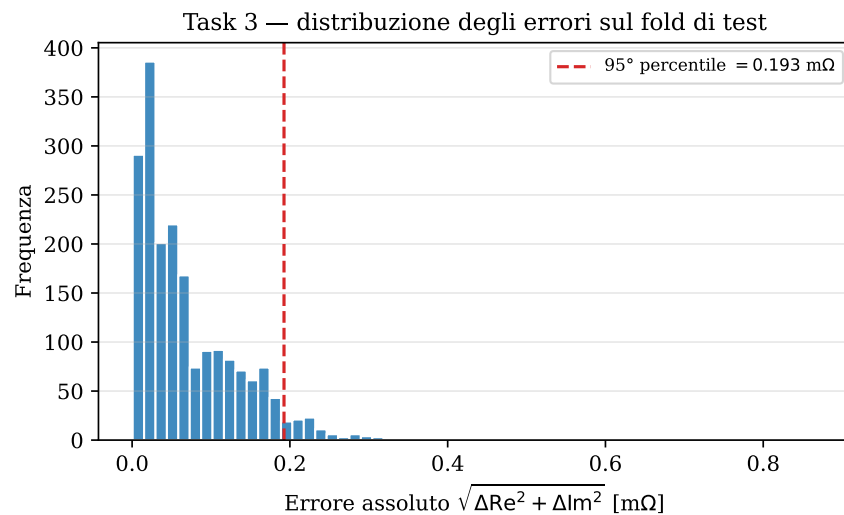
Figura 7.4: Istogramma degli errori assoluti \sqrt{\Delta \text{Re}^2 + \Delta \text{Im}^2} sul fold di test. Il 95° percentile cade sotto i 0.2 mΩ, ben dentro la dispersione fisiologica delle misure.
