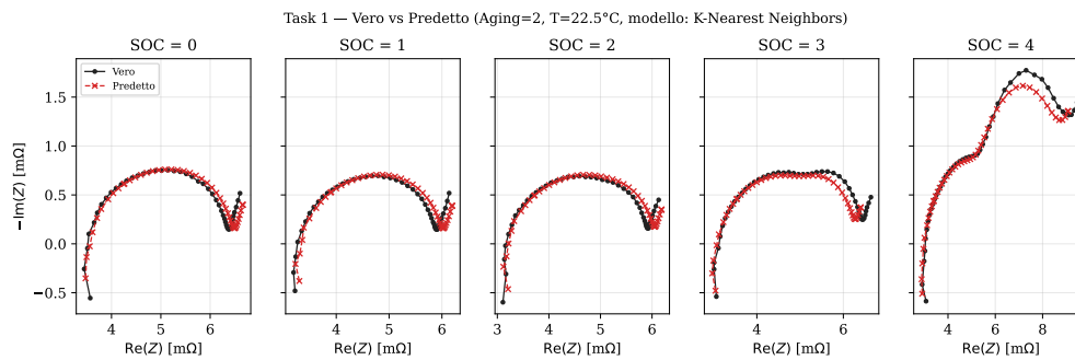
Figura 5.2: Curve previste (rosso, tratteggiate) sovrapposte alle vere (nero) per la coppia ( Aging = 2, T = 22.5^\circ C ) esclusa, una per ciascuno dei 5 livelli di SOC. Il modello vincente (KNN distance-weighted) ricostruisce semicerchio e coda diffusiva con errore inferiore al millesimo di milliohm.
