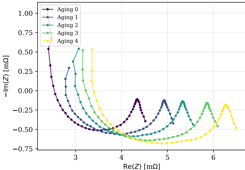
Evoluzione delle curve di Nyquist con l'invecchiamento ( T = 25\text{ }^{\circ}\text{C} , \text{SOC} = 2 )
