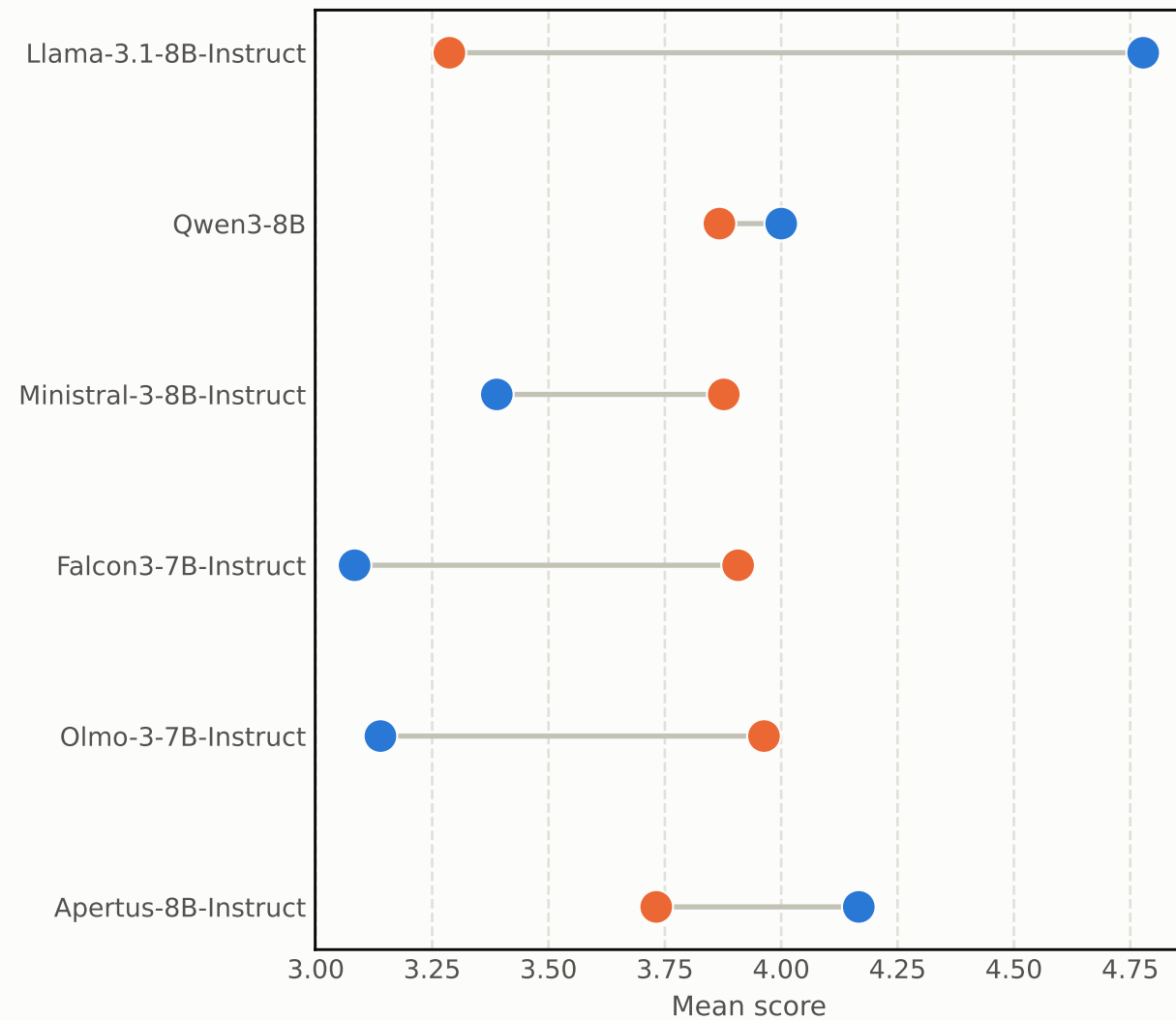
MFT
