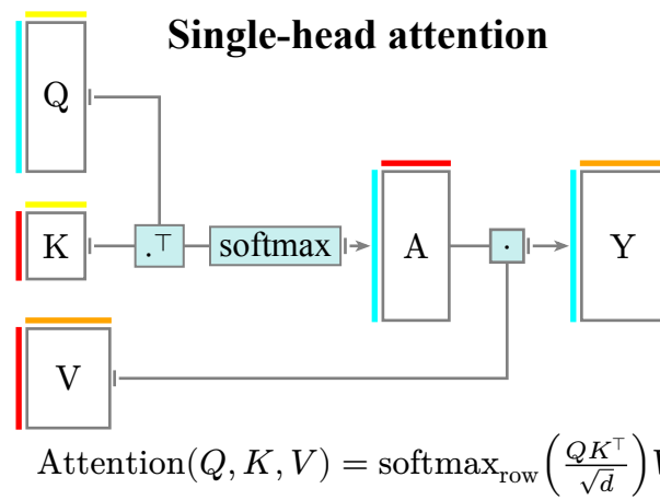
Abbildung 2: Attention Diagram
