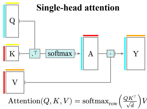
Abbildung 2: Attention Diagram
