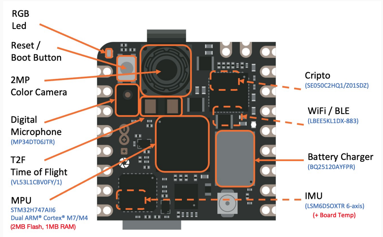
Arduino Nicla Vision
