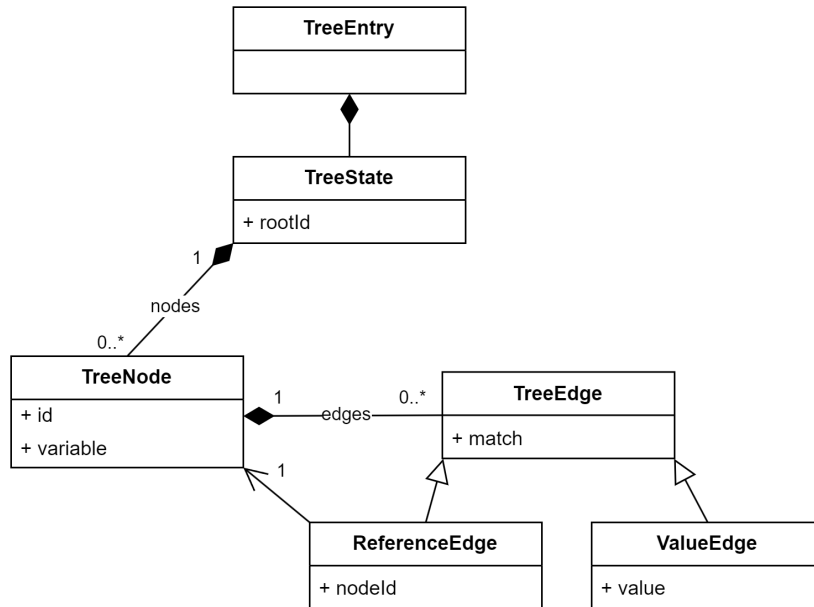
Obr. 3.15: Triedny diagram pre editor interpretácií funkcií.
