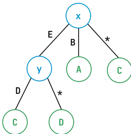
Obr. 3.9: Všeobecný strom pre Editor interpretácií funkcií rozborom prípadov.
