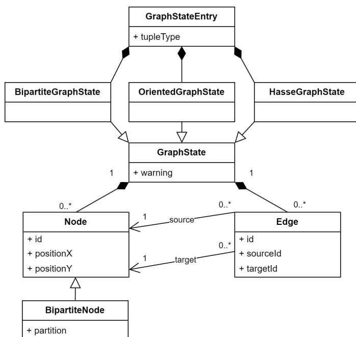
Obr. 3.14: Triedny diagram pre grafové editory.
