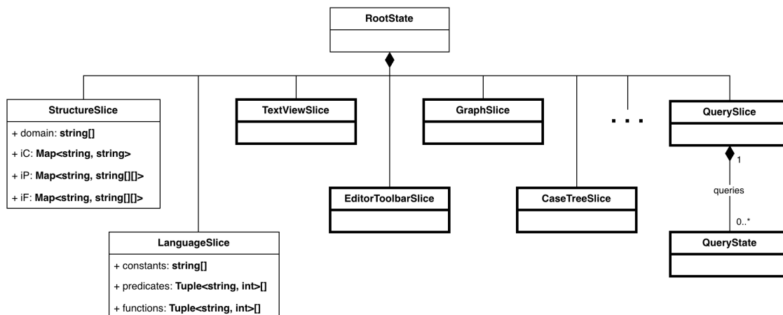
Obr. 3.14: Triedny diagram vybraných súčastí stavu aplikácie.
