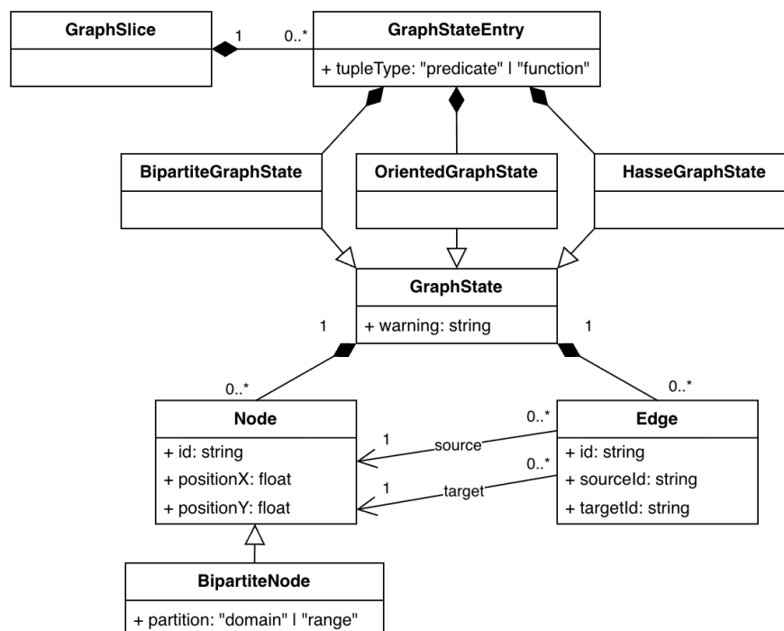
Obr. 3.15: Triedny diagram pre grafové editory.
