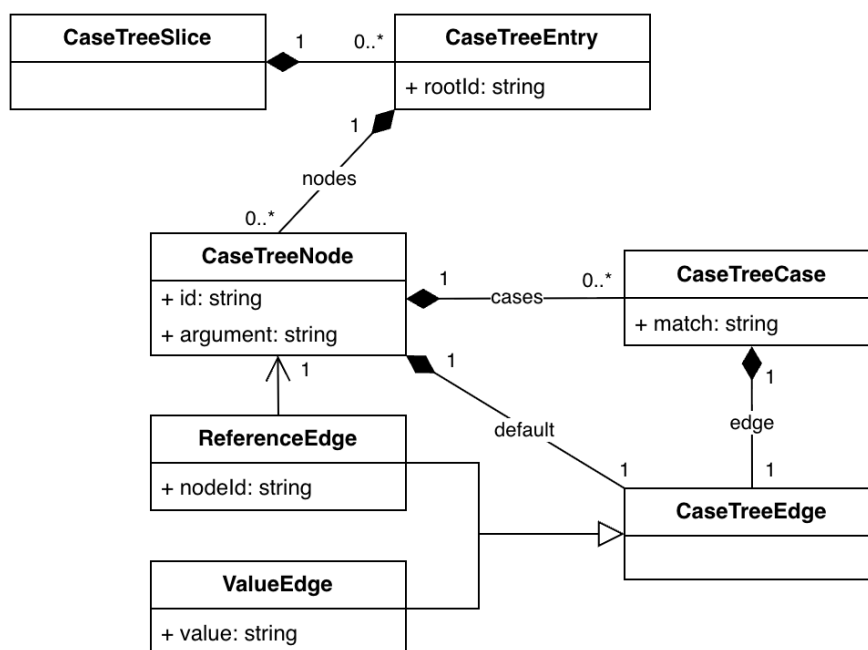
Obr. 3.16: Triedny diagram pre editor interpretácií funkcií rozborom prípadov.
