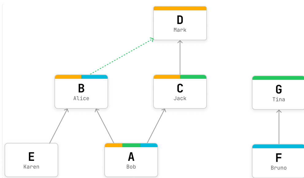
Obr. 3.5: Návrh vizuálu pre Hasseho diagram.
