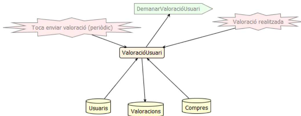
Fig. 36 Enregistrador de valoracions Agent Overview Diagram
