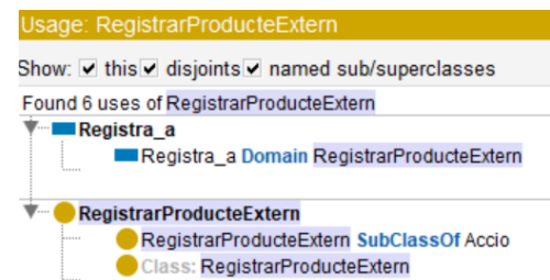
Fig. 53 Usage ResgistrarProducteExtern
