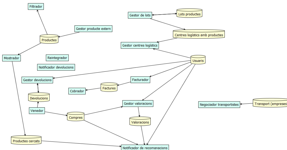
Fig. 22 Data Coupling
