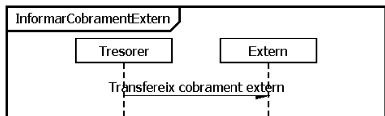
Fig. 29 Protocol InformarCobramentExtern
