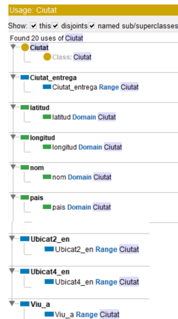
Fig. 58 Usage Ciutat
