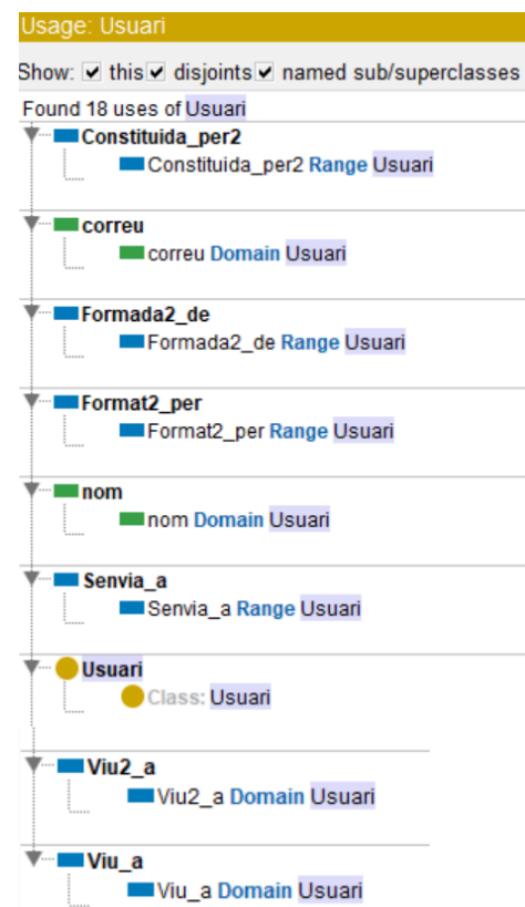
Fig. 70 Usage Usuari
