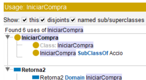
Fig. 51 Usage IniciarCompra
