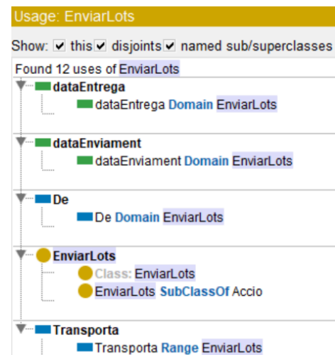
Fig. 50 Usage EnviarLots
