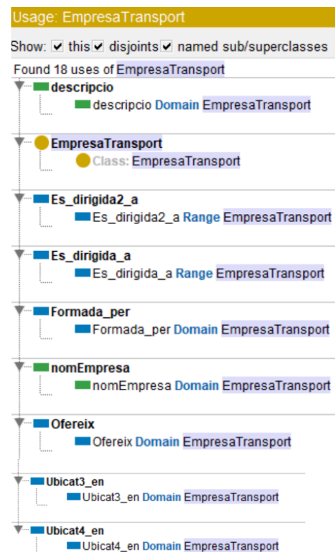
Fig. 62 Usage EmpresaTransport
