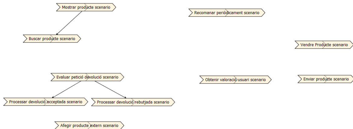
Fig. 2 Scenarios
