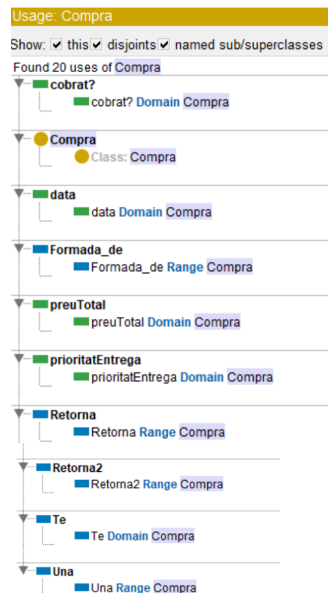
Fig. 59 Usage Compra
