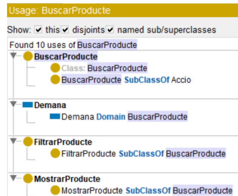
Fig. 47 Usage BuscarProducte
