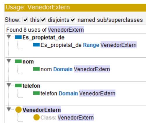
Fig. 72 Usage VenedorExtern
