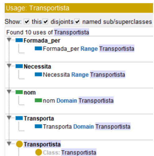
Fig. 69 Usage Transportista
