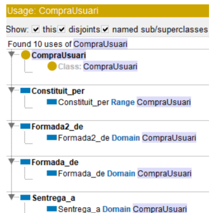
Fig. 60 Usage CompraUsuari
