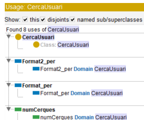
Fig. 57 Usage CercaUsuari
