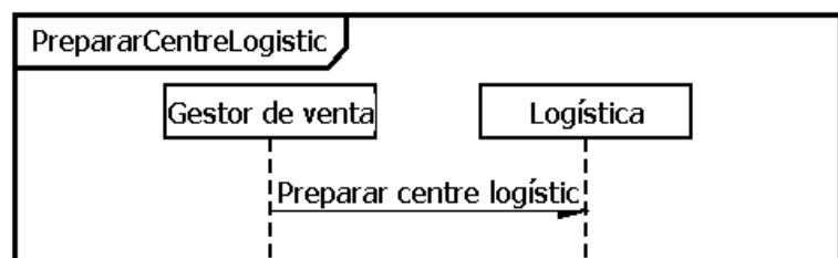
Fig. 26 Protocol PrepararCentreLogístic
