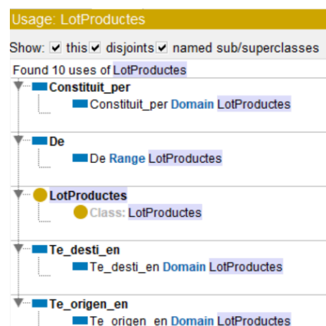
Fig. 63 Usage LotProductes
