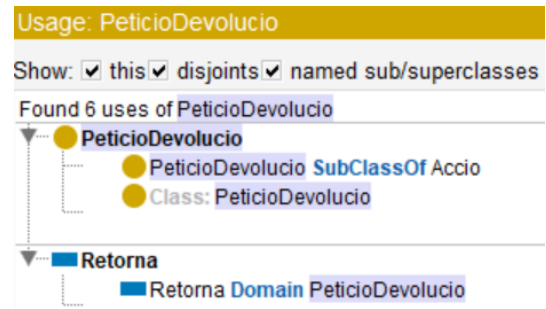
Fig. 52 Usage PeticioDevolucio
