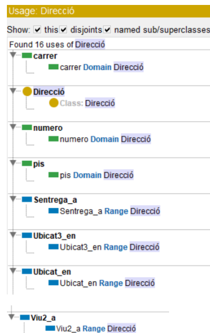
Fig. 61 Usage Direcció
