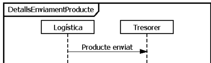
Fig. 28 Protocol DetallsEnviamentProducte
