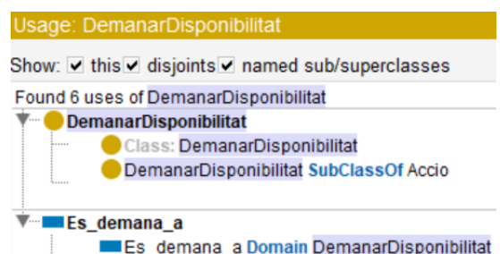
Fig. 48 Usage DemanarDisponibilitat
