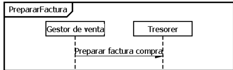
Fig. 27 Protocol PrepararFactura
