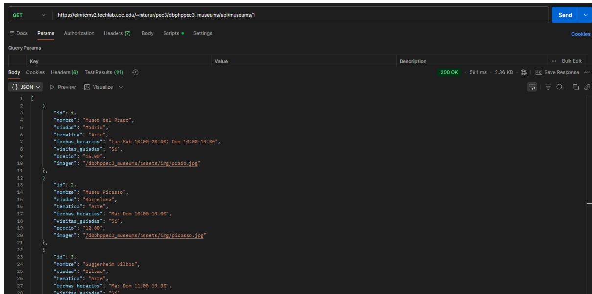
Fig. 13 - Consulta de API_museums (página 1) desde POSTMAN.
