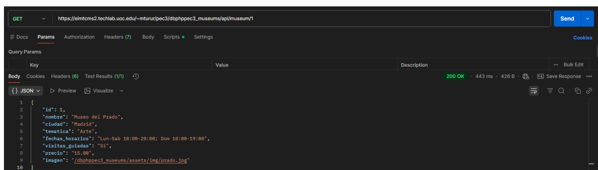
Fig. 14 - Consulta de API_museum (id del museo 1) desde POSTMAN.
