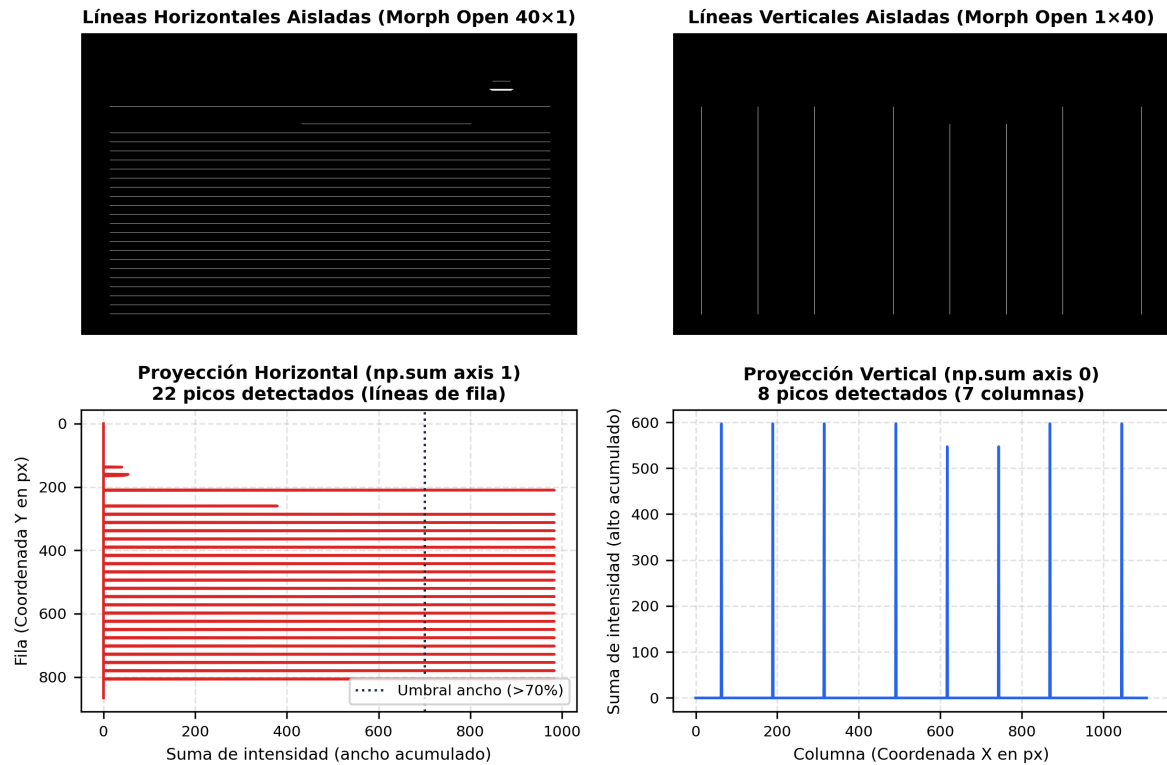
Figura 3: Detección estructural de tabla: Líneas aisladas con Morph Open (40x1 y 1x40) y perfiles de proyección 1D (axis 1 y axis 0).
