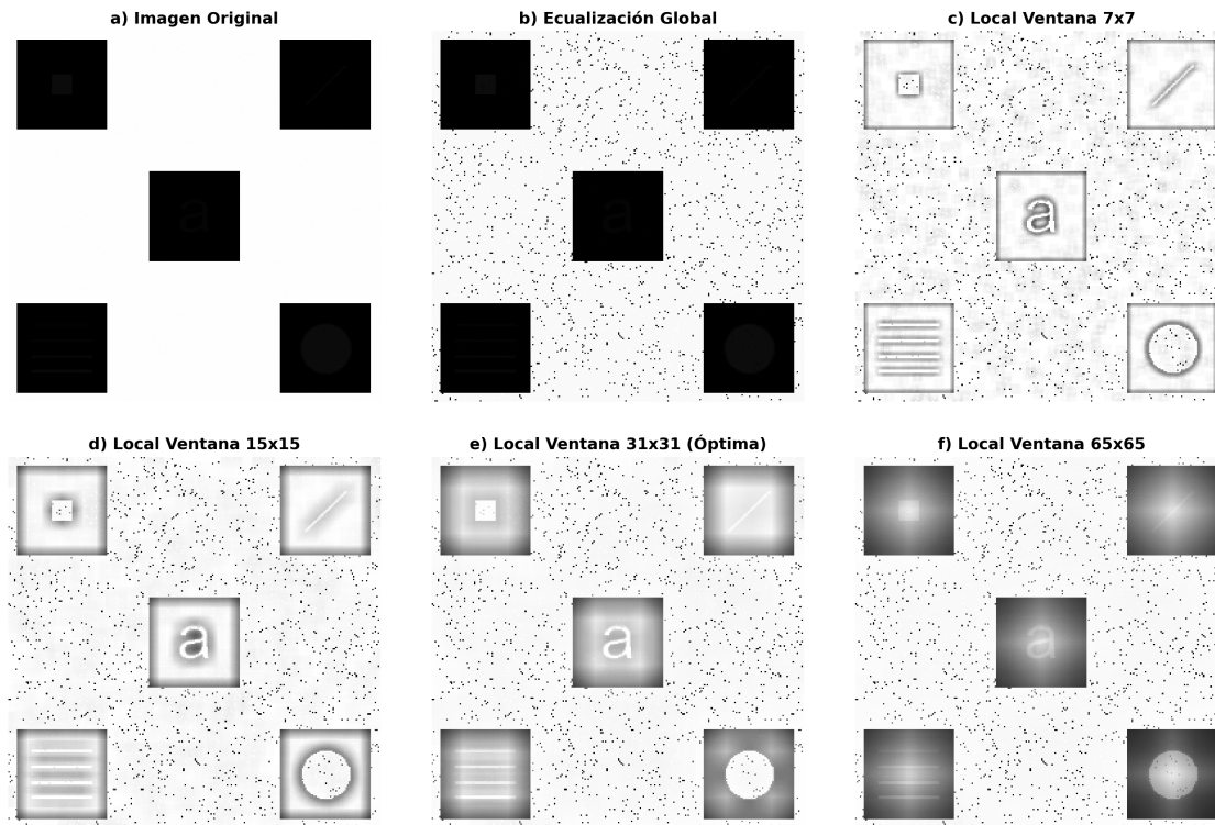
Figura 1: Comparativa visual con proporciones geométricas cuadradas (1:1): a) Original, b) Global, c-f) Ventanas de 7×7 a 65×65.
