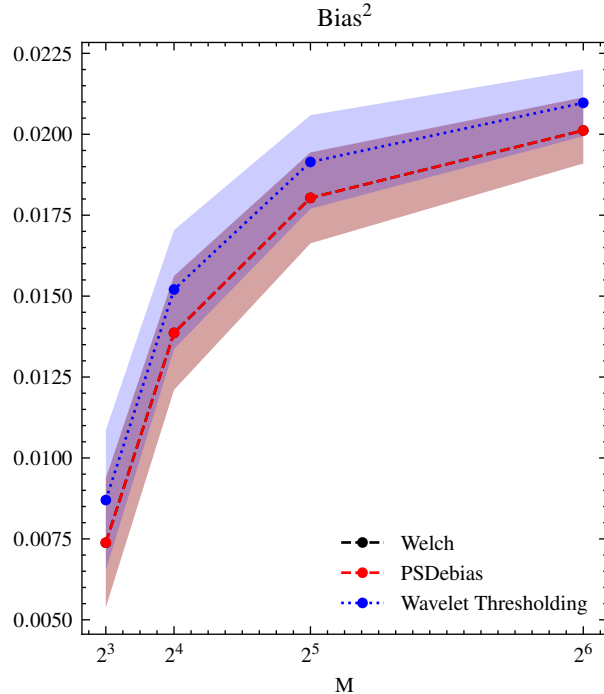
Matérn
