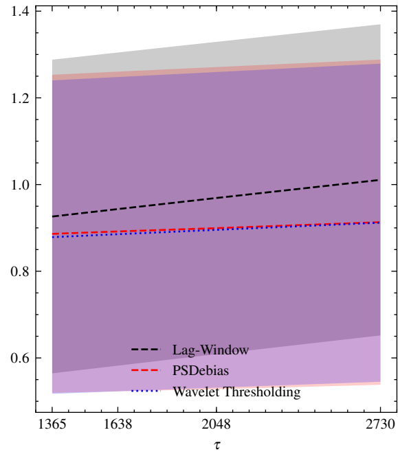
Var
