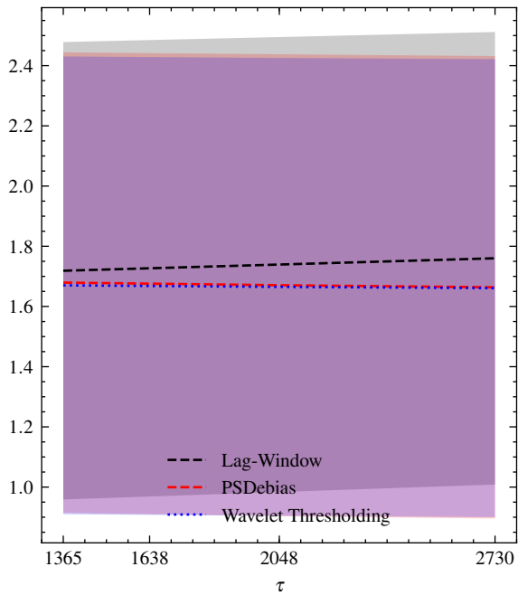
MSE
