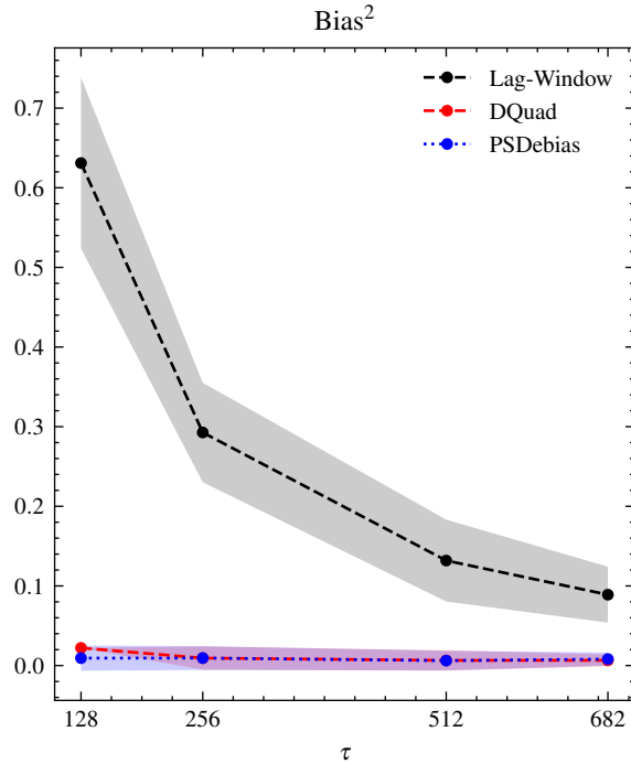
Matérn
