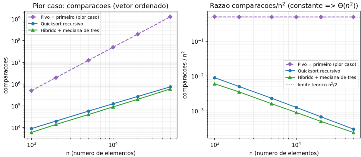
Figura 7 – Pior caso: número de comparações e razão comparações/ n^2 .
