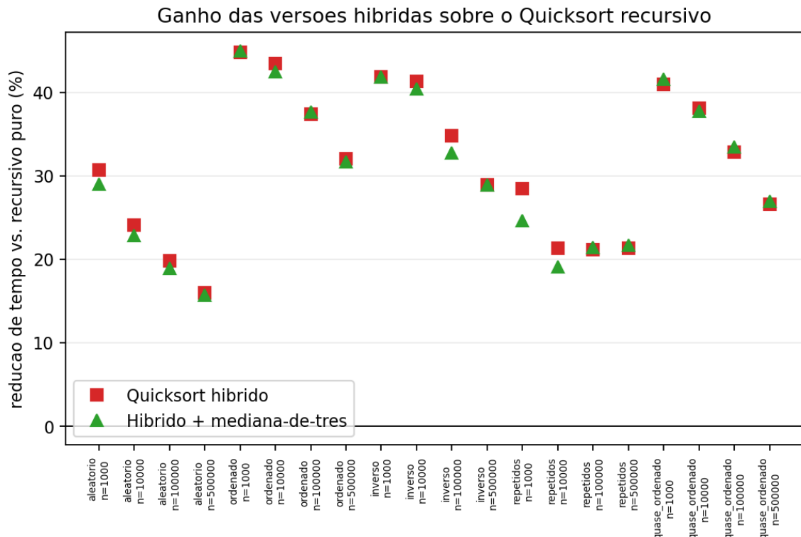
Figura 6 – Redução do tempo de execução das versões híbridas em relação ao Quicksort recursivo.
