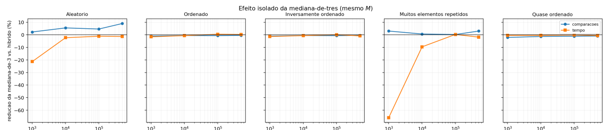
Figura 7 – Efeito isolado da mediana-de-três, ambos com M = 40 : redução percentual das comparações e do tempo em relação ao híbrido simples. Valores positivos indicam vantagem da mediana-de-três.
