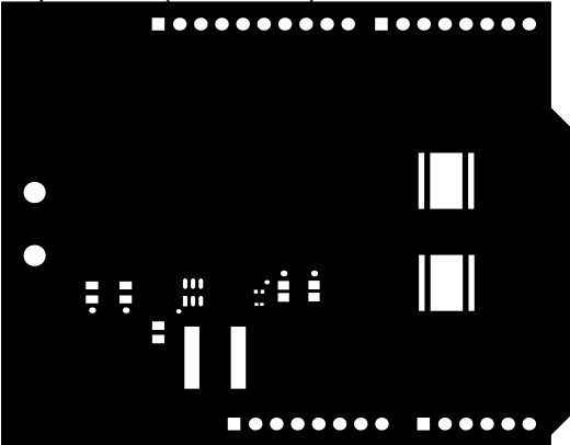
Top Solder (Scale: 1:1)
