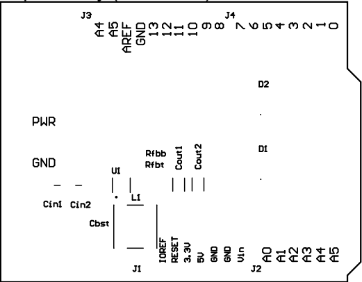
Top Overlay (Scale: 1:1)
