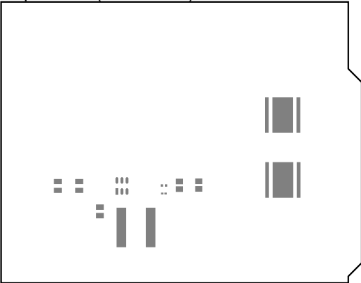
Top Paste (Scale: 1:1)
