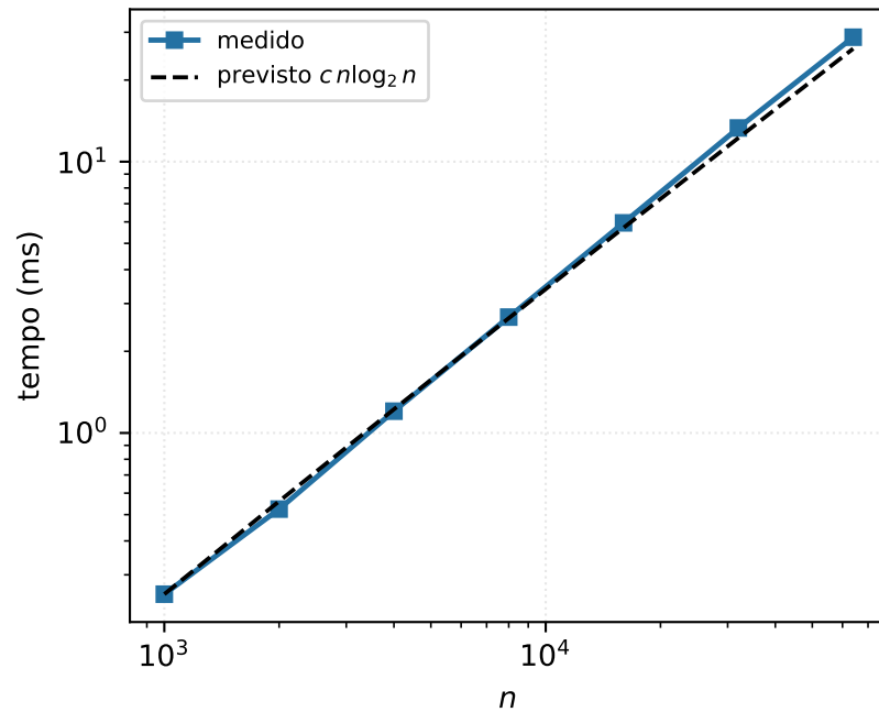
Dijkstra Heap Mínimo ( O(n \log n) )
