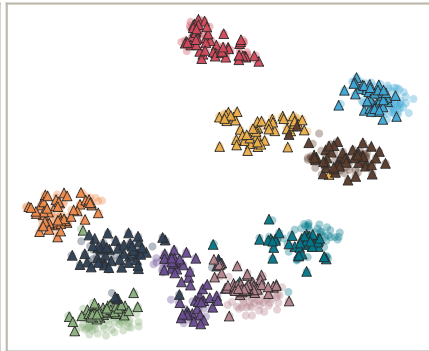
CLIP ViT-B/32
