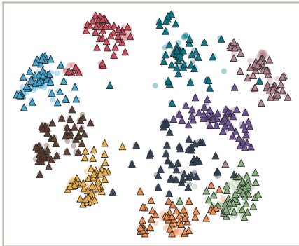
ViT-B/16
