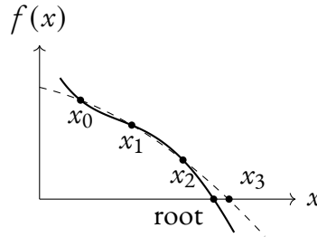
Fig. 1.5: iteration muller
