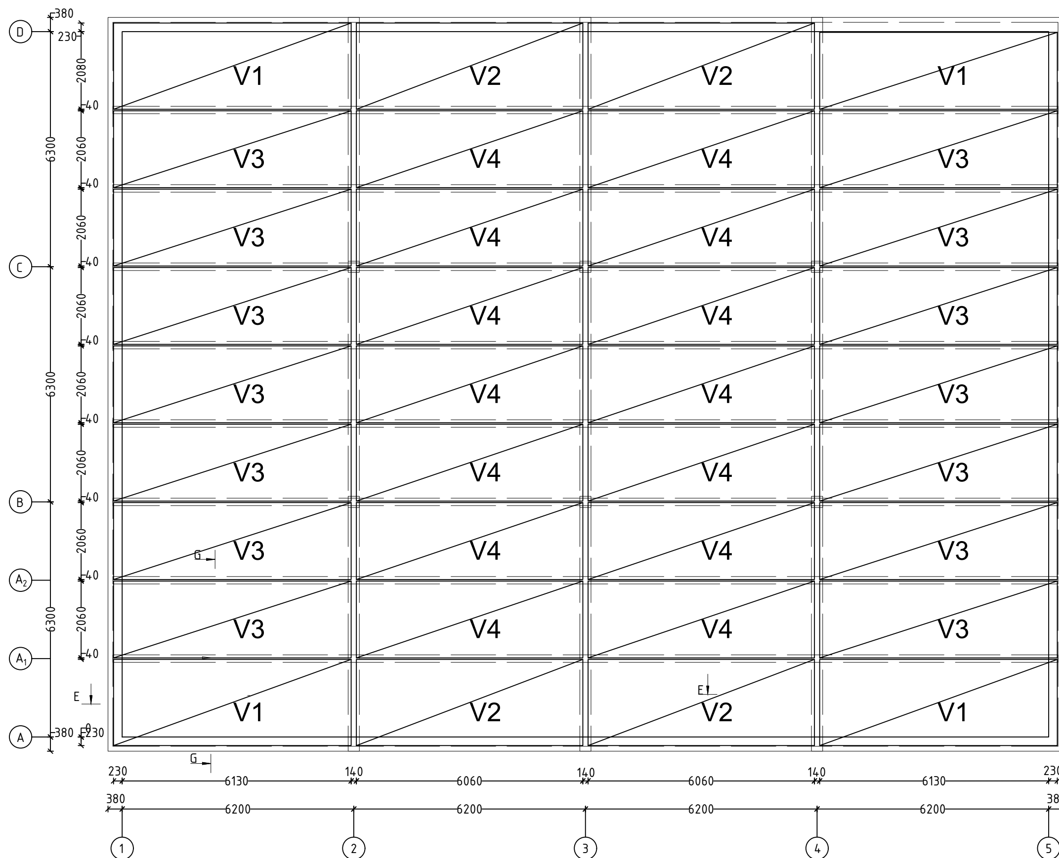
VAHELAEPLAADI ALUMISE PINNA ARMEERING 1:100
