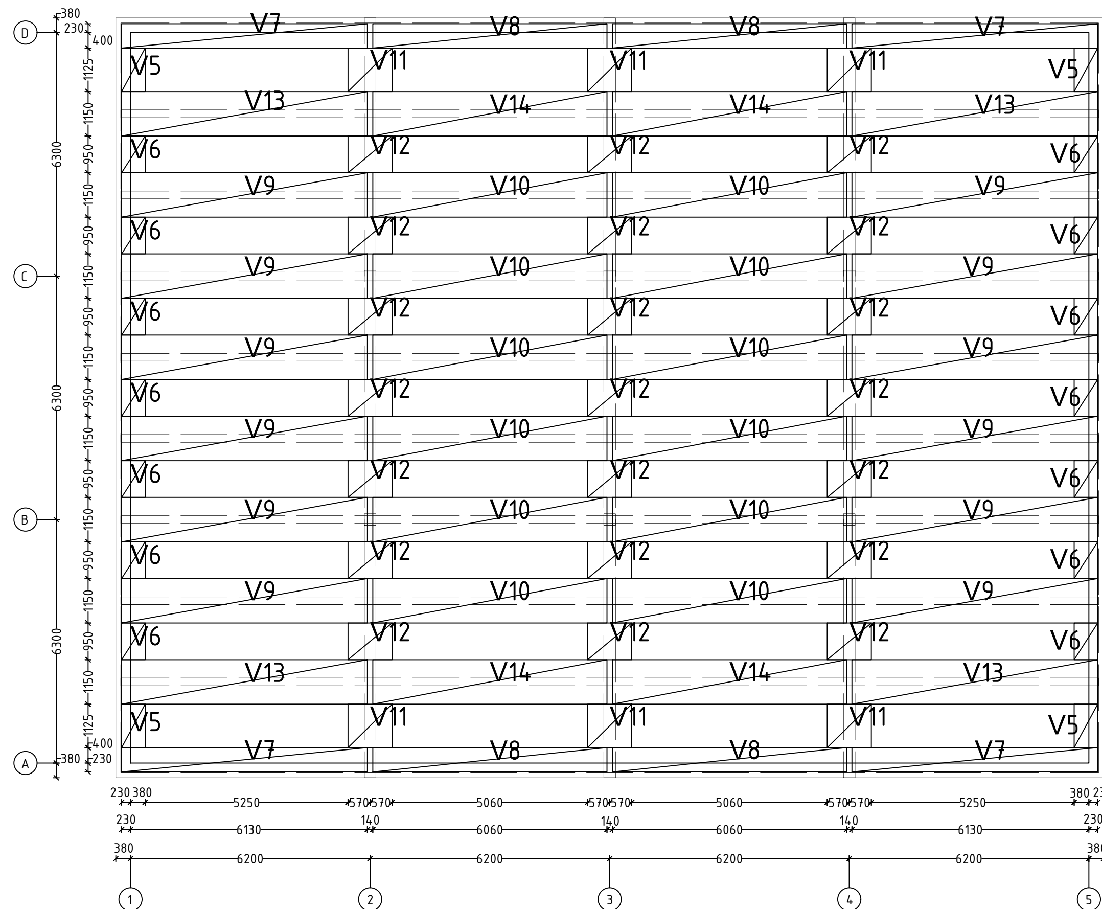
VAHELAEPLAADI ÜLEMISE PINNA ARMEERING 1:100
