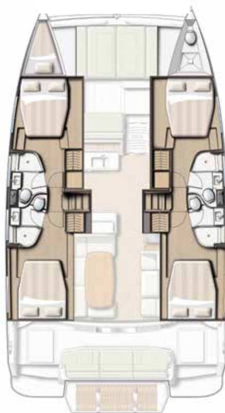
KABINA ZAŁOGI (OPCJA)
