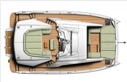
UKŁAD ARMATORSKI
