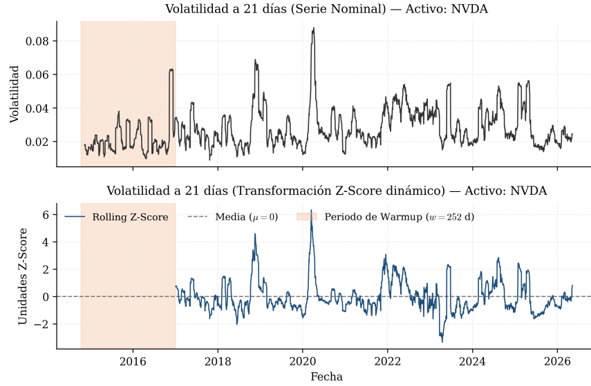
Figura 9: Evolución de la volatilidad para el activo NVDA. Arriba: Serie nominal. Abajo: Serie tras la aplicación del Z-Score dinámico y convergencia hacia la media móvil ( \mu = 0 ). El área sombreada denota el periodo de warmup (calentamiento). Fuente: Elaboración propia.
