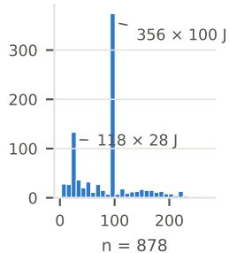
Énergie Charpy
