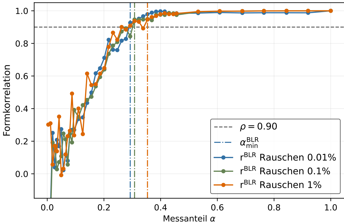
Formkorrelation der BLR-Rekonstruktion für verschiedene Rauschen
