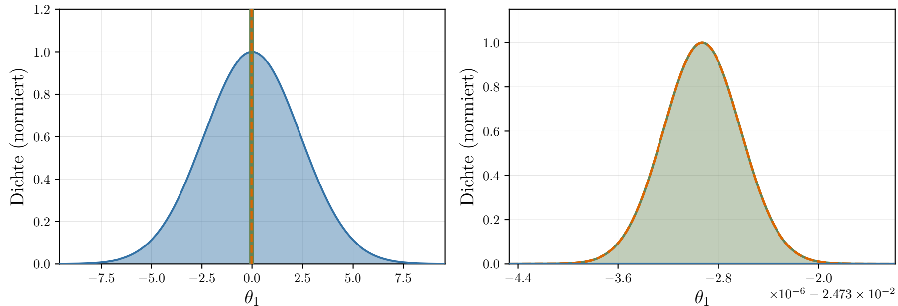
Bayes Update des DCT Koeffizienten \theta_1 bei \alpha_{\min}^{\text{BLR}} = 0.293 (Rauschen 0.01%, k = 77 )
