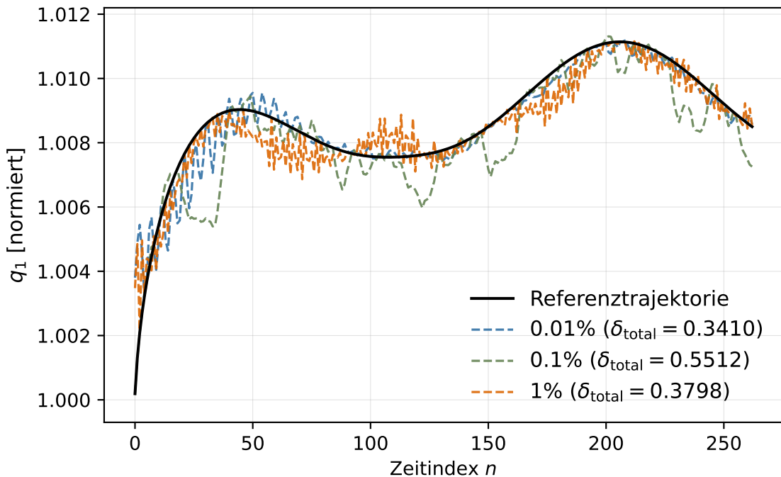
q_1 über der Zeit bei \alpha_{\min}^{\text{CS}}
