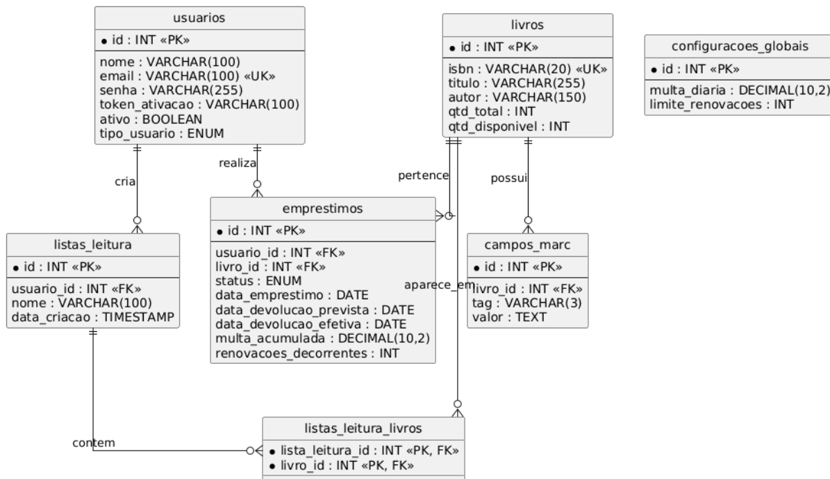
Figura 2: Diagrama Entidade-Relacionamento do banco de dados
