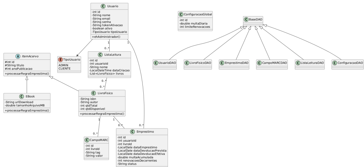
Figura 1: Diagrama de Classes do sistema Biblioteca MARC21
