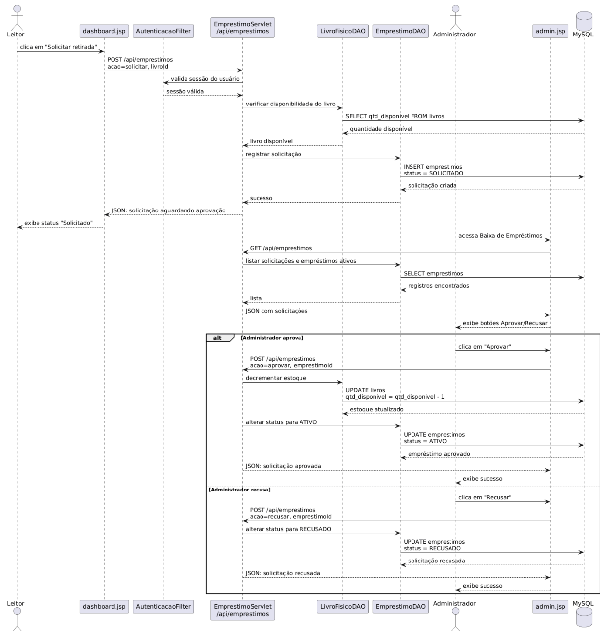
Figura 4: Diagrama de Sequência: solicitação e aprovação de empréstimo
