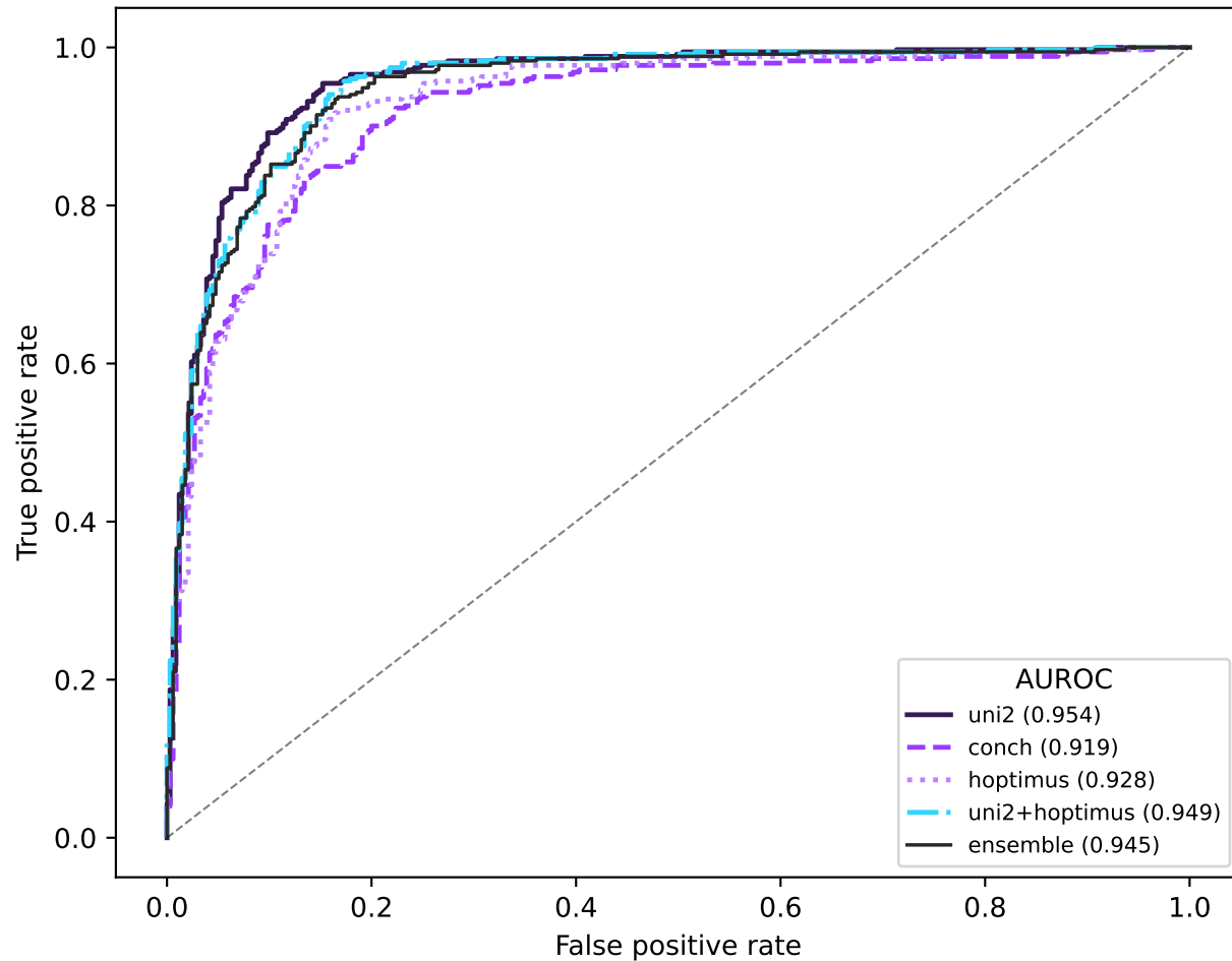
ROC
