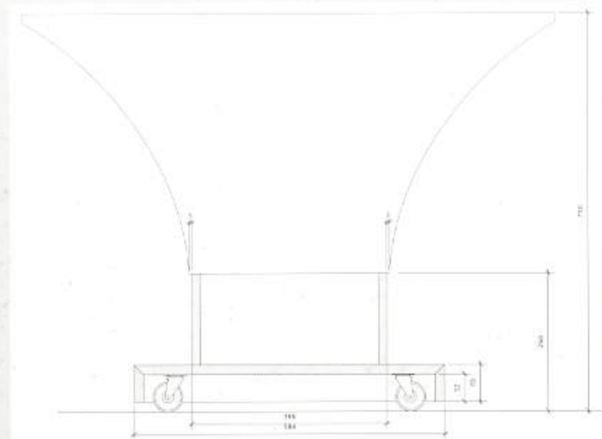
Sección de una de las mesas móviles
