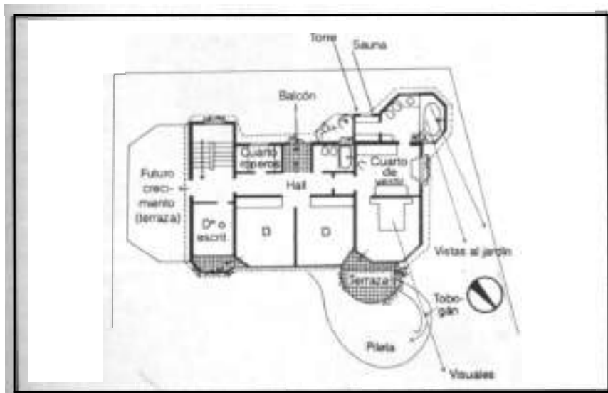
Planta alta. Tobogán para tirarse a la pileta desde la terraza del dormitorio de los padres.
