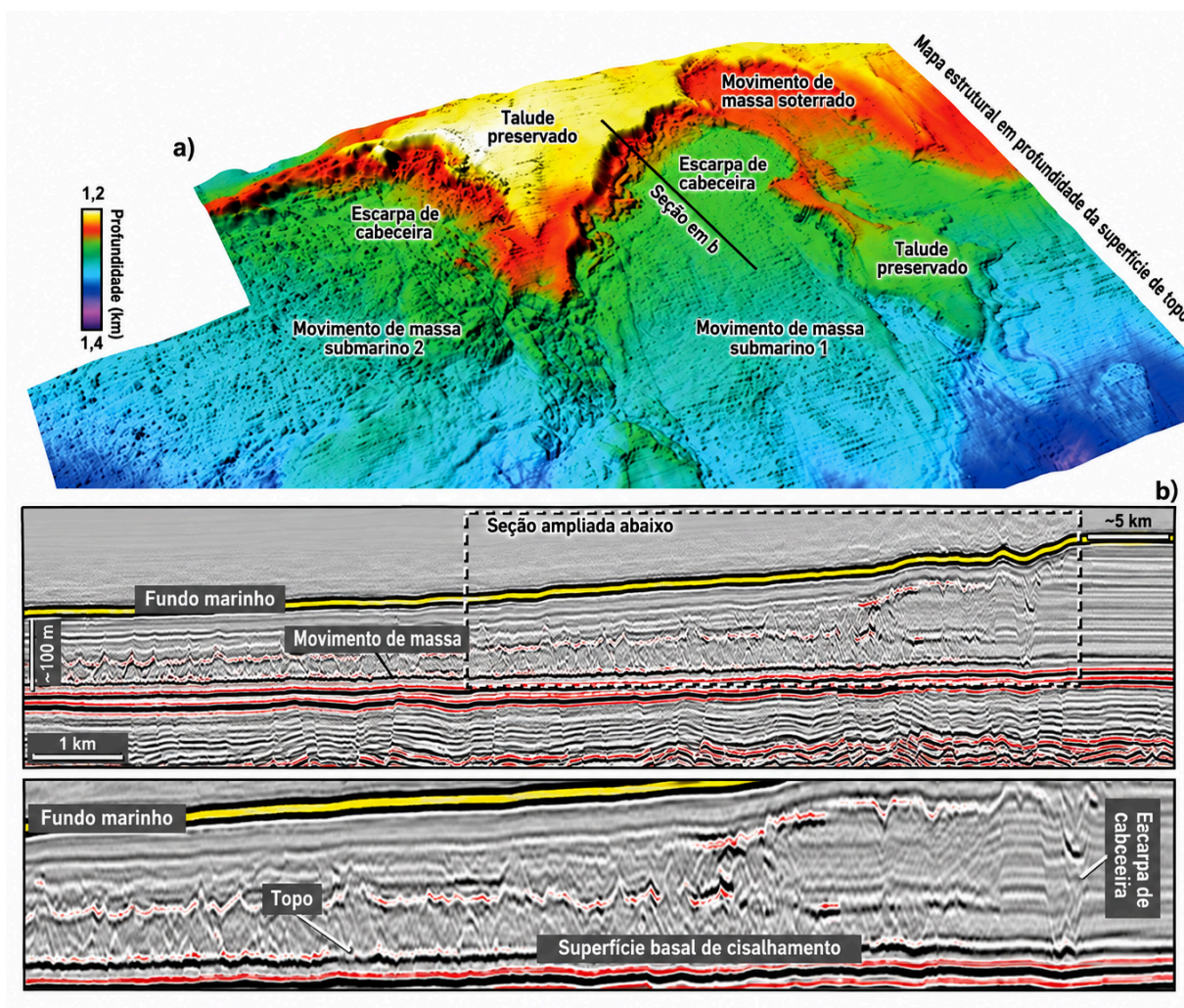
Figura 9 — Exemplo de movimento de massa submarino em dados de sísmica de reflexão: (a) mapa estrutural da superfície de topo, com a distribuição do depósito e as escarpas de cabeceira; (b) seção sísmica vertical, com a superfície de topo, a superfície basal de cisalhamento e a massa sedimentar deformada.
