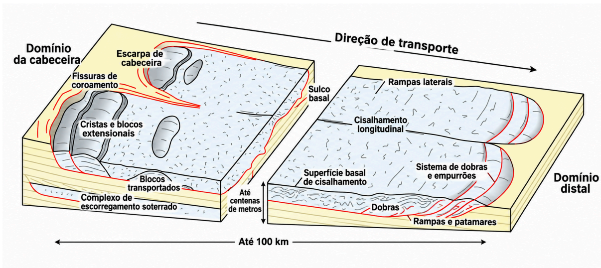
Figura 12 — Ilustração esquemática da morfologia e das estruturas de um movimento de massa submarino.
