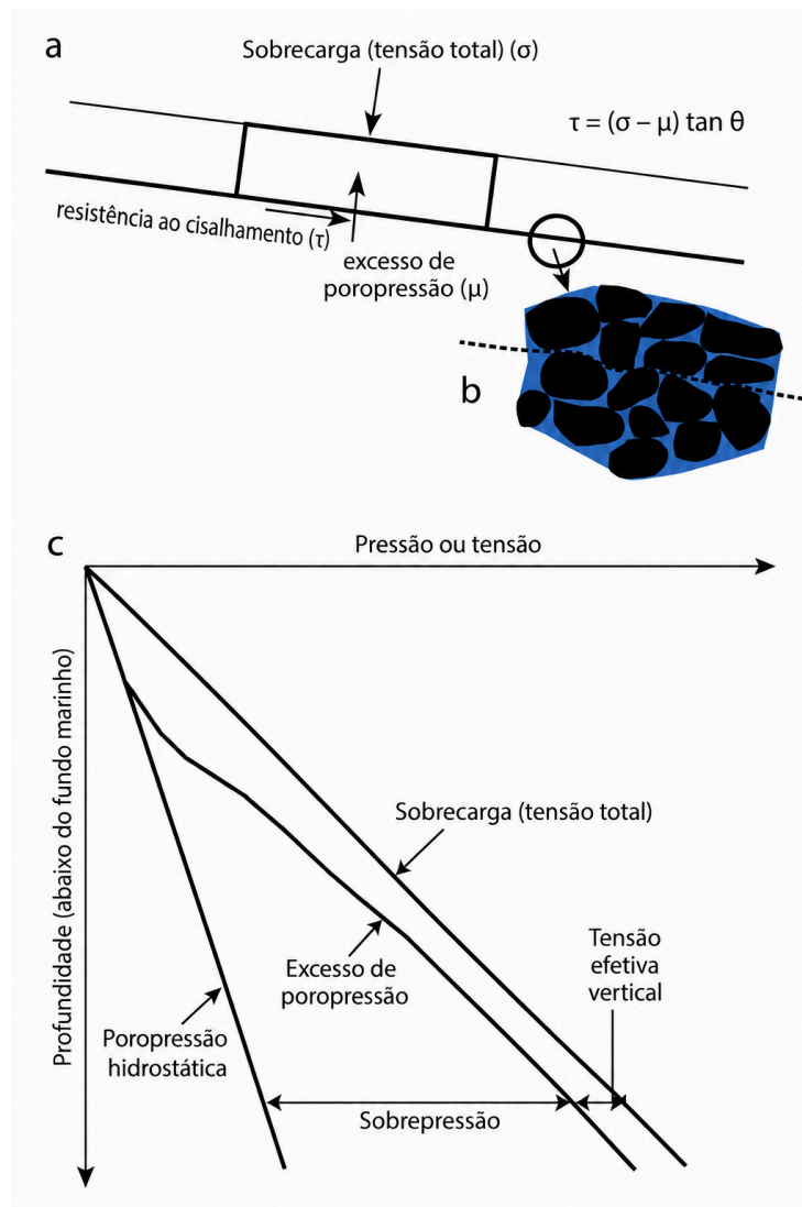
Figura 5 — Relações entre tensão total, poropressão, tensão efetiva e resistência ao cisalhamento em sedimentos marinhos saturados
