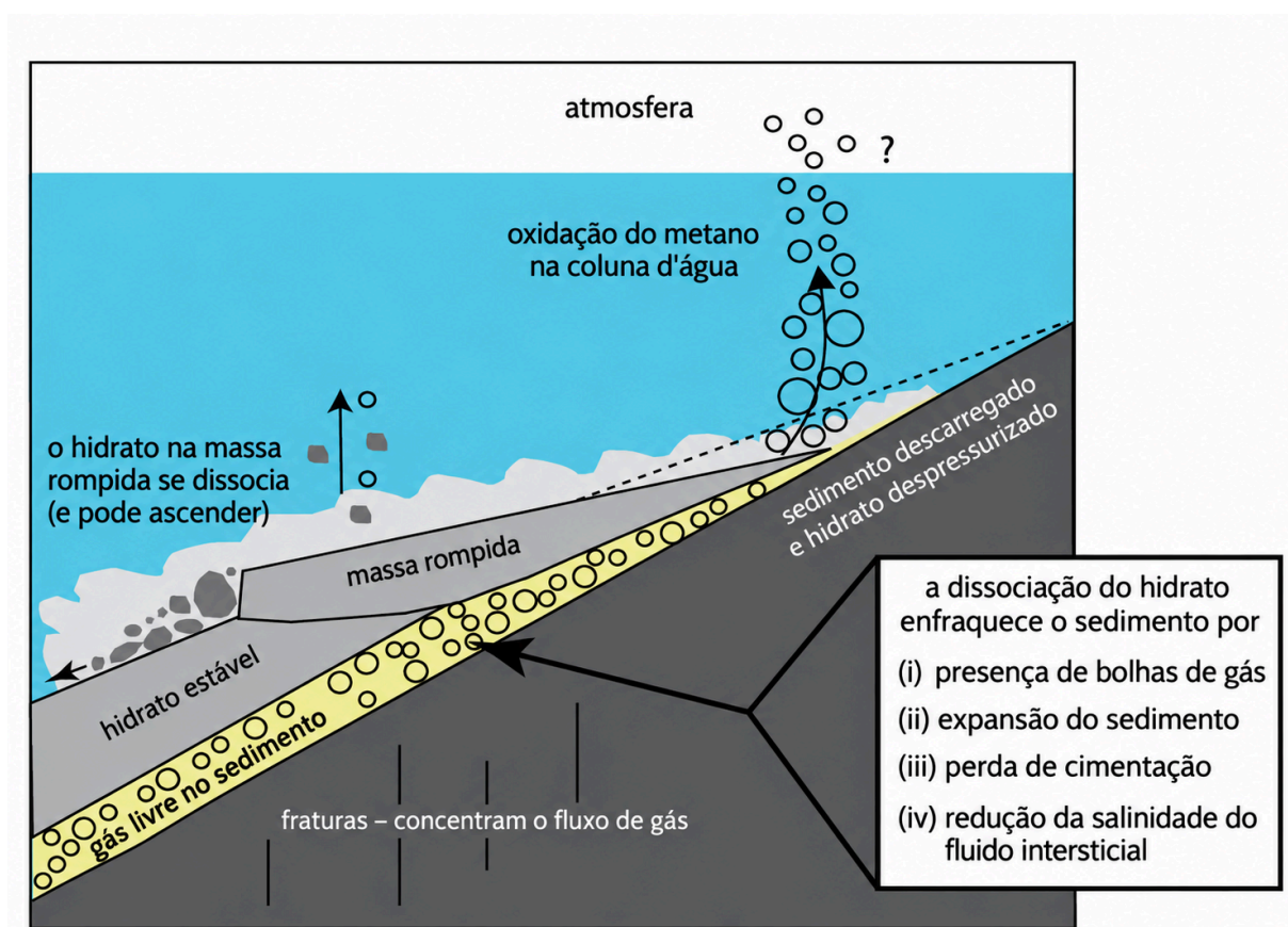
Figura X – Síntese dos processos de dissociação de hidratos de gás previamente propostos como possíveis causas de movimentos de massa submarinos ou de emissões de metano.
