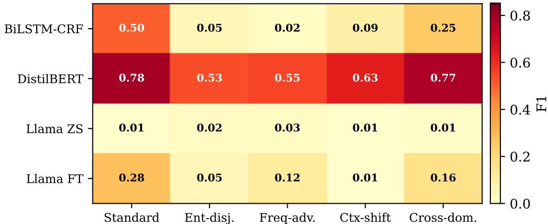
Span-level F1 heatmap
