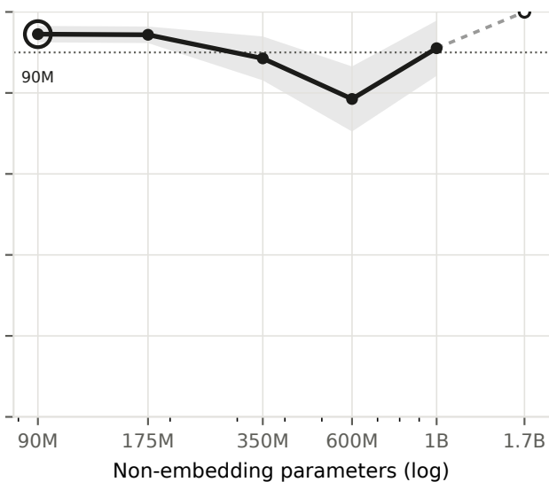
BPB
