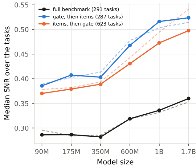
SNR
