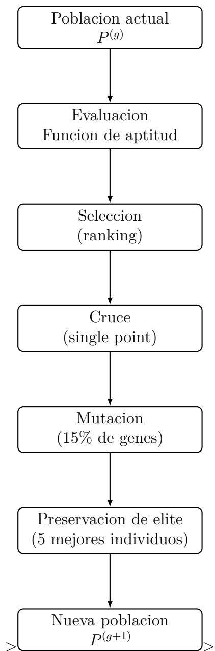
Figure 5.2: Flujo del ciclo evolutivo del algoritmo genetico en PyGAD.
