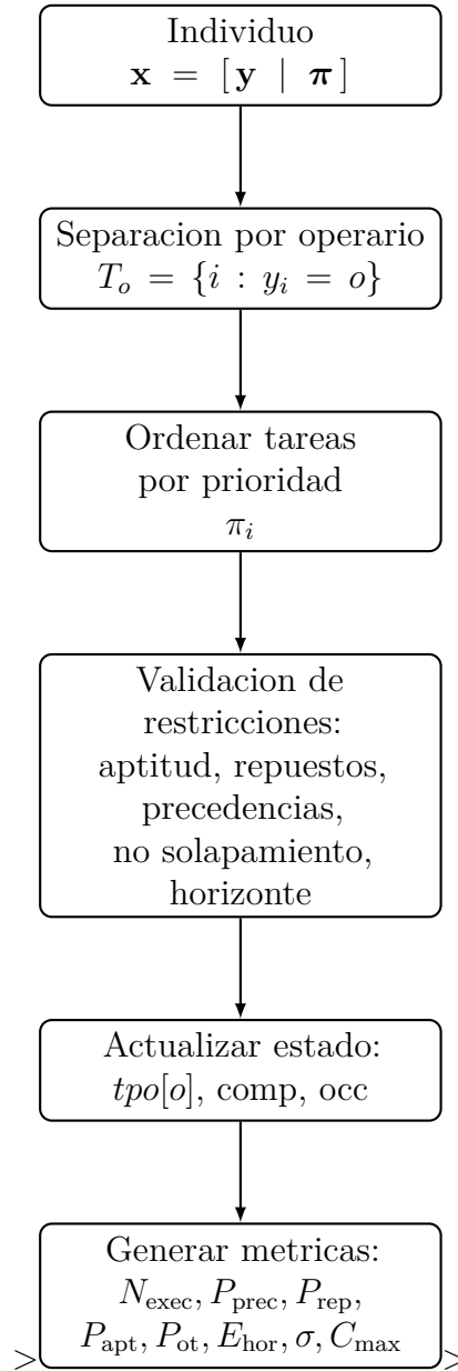
Figure 5.1: Flujo del proceso de evaluacion de un individuo.
