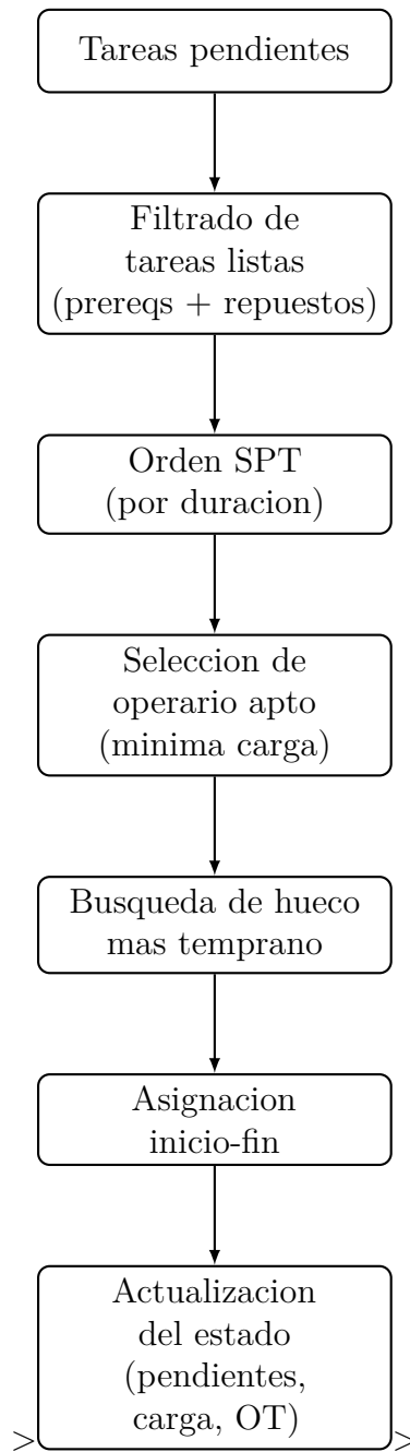
Figure 5.3: Flujo operativo del metodo SPT en el taller.
