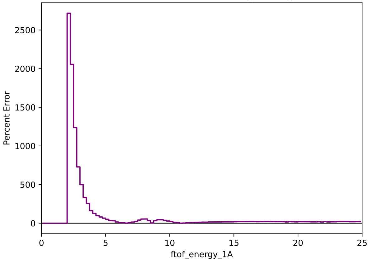
Percent Error: Data vs MC (ftof_energy_1A)
