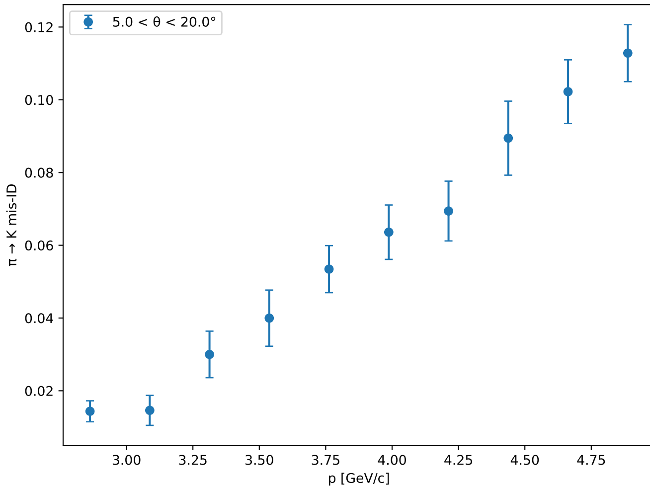
\pi \rightarrow K Mis-ID vs Momentum
