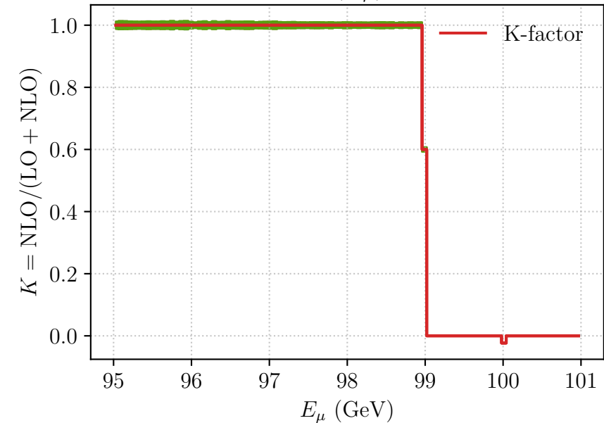
K(E_\mu)
