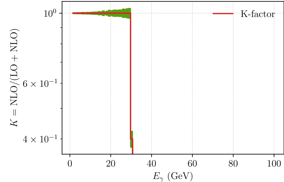
K(E_\gamma)
