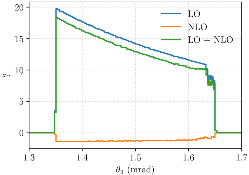
Muon Scattering Angle
