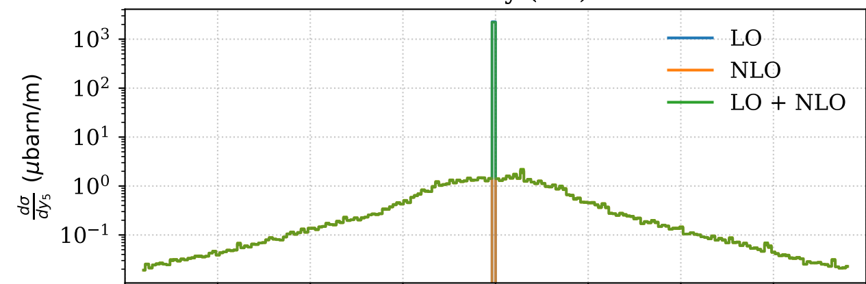
Photon y(lab)
