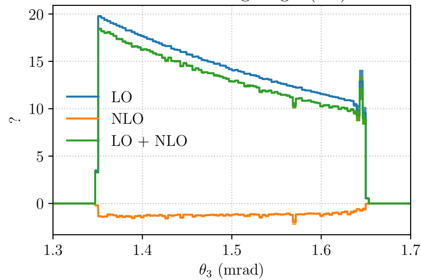
Muon Scattering Angle (lab)
