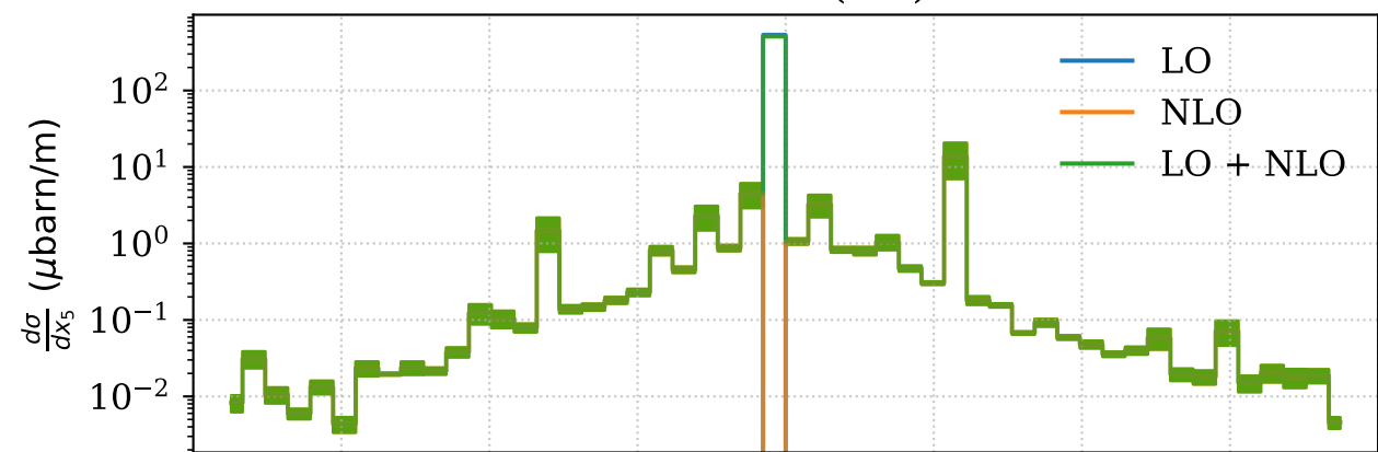
Photon x(lab)
