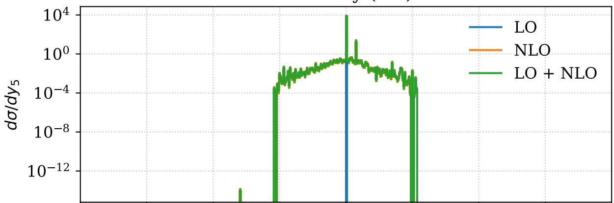
Photon y(lab)
