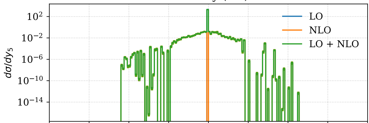
Photon y (lab)
