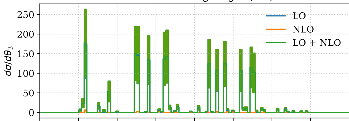
Muon Scattering Angle (lab)
