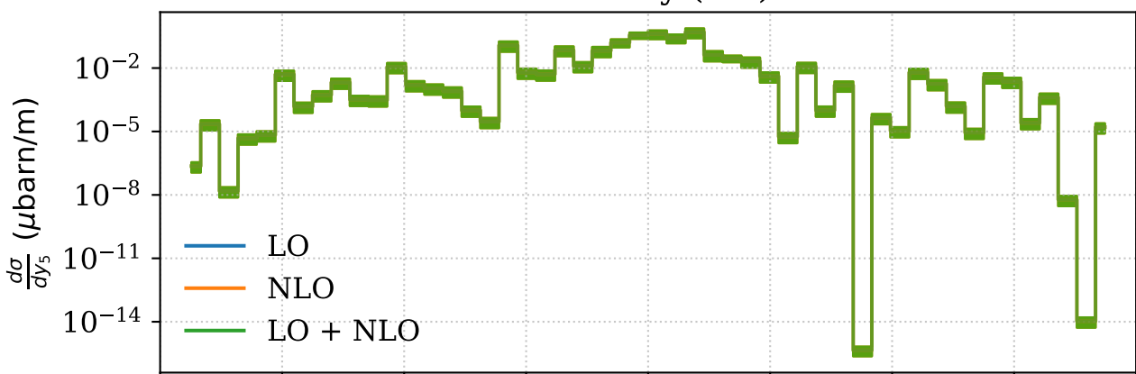
Photon y(lab)
