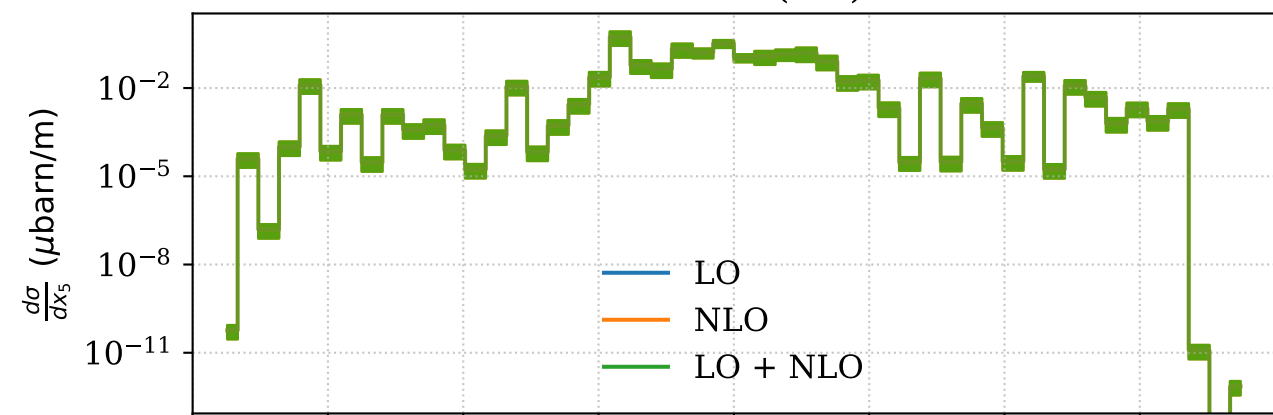
Photon x(lab)
